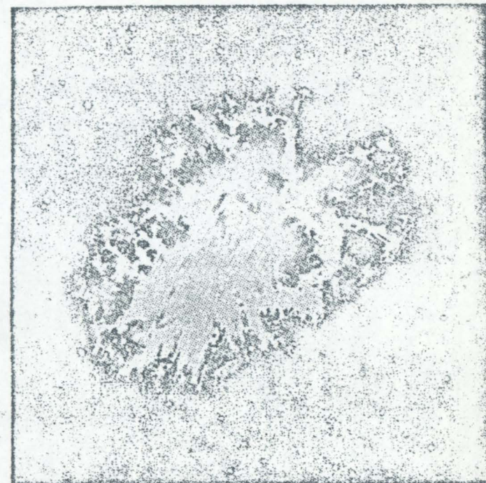
Krabbnubulosa, vars kärna består av neutronstjärnor av oerhört stor täthet roterar mycket snabbt. Teoretiskt kan den i sin periferi ha högre hastigheter än ljuset
